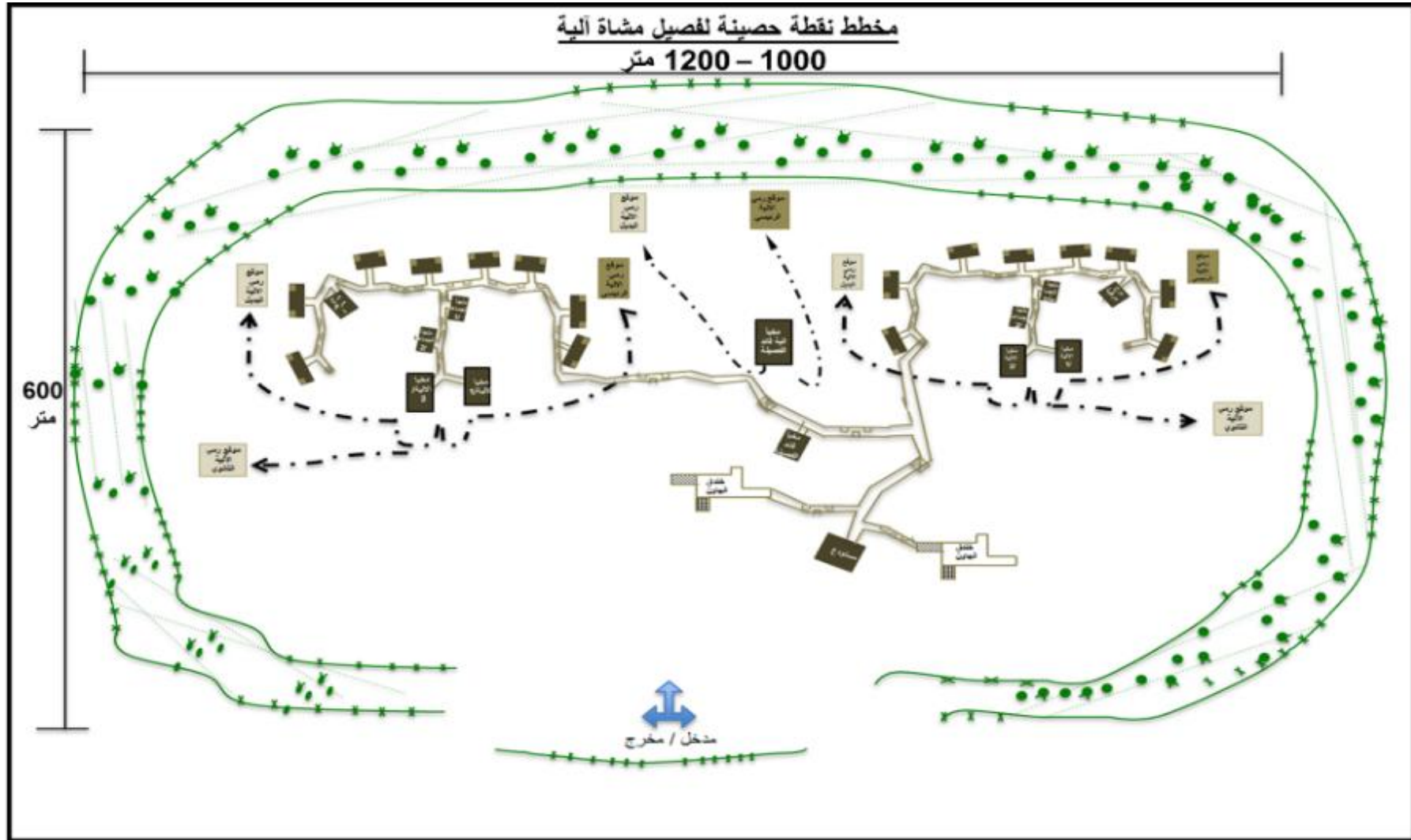
الشكل رقم (26) مخطط نقطة حصينة لفصيل مشاة آلية
